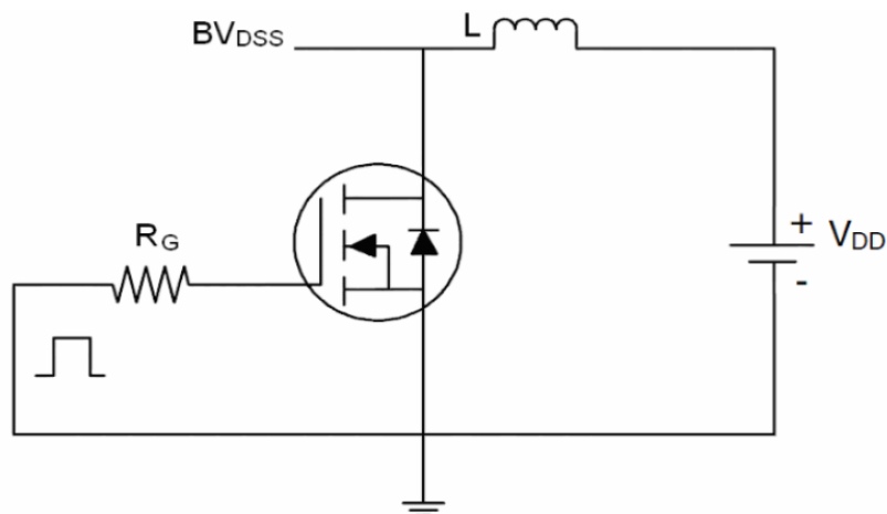
1) E_{AS} TEST CIRCUIT
